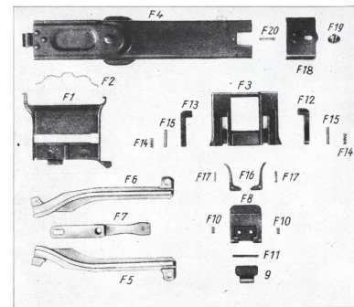
MG 34, Einzelteile: Zuführer und Zuführerdeckel
