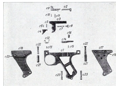
MG 34, Einzelteile: Griffstück
